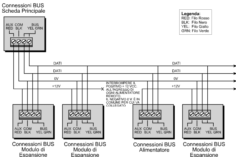
Figura 2-3: Espansione BUS a 4 fili
