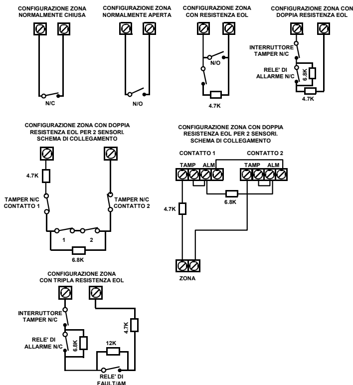
Figura 2-4: Schema di Collegamento delle Zone
