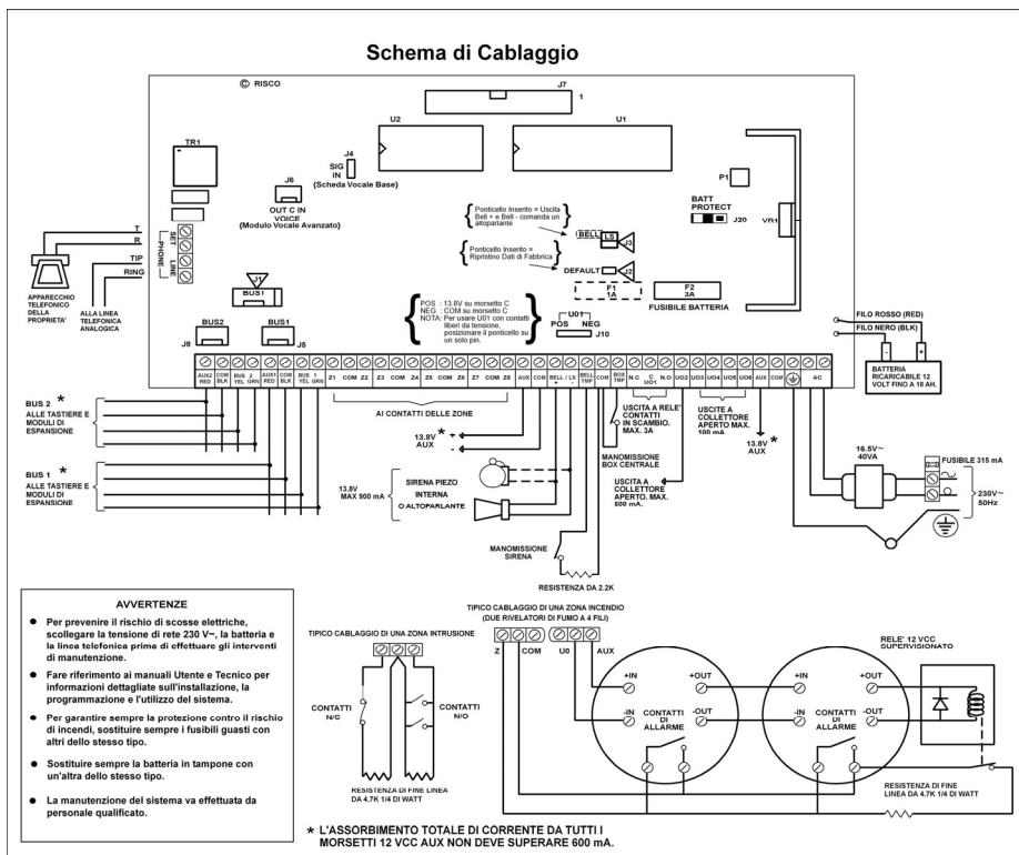
Figura 2-2: Schema di Cablaggio della Scheda Principale.
