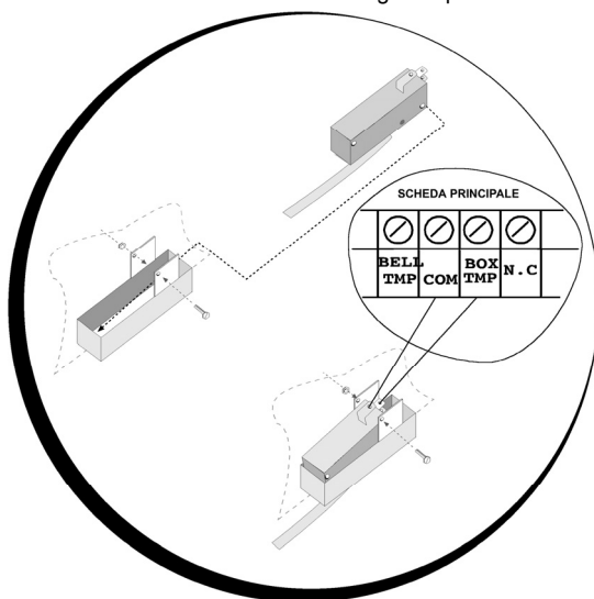
Figura 2-5: Cablaggio del Tamper del Contenitore metallico
