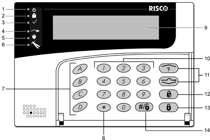
Figura 4-1: Tastiera LCD
