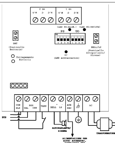
Figure 3-9: Modulo di Espansione Alimentazione 3A (Esempio di Cablaggio dell'alimentatore)
