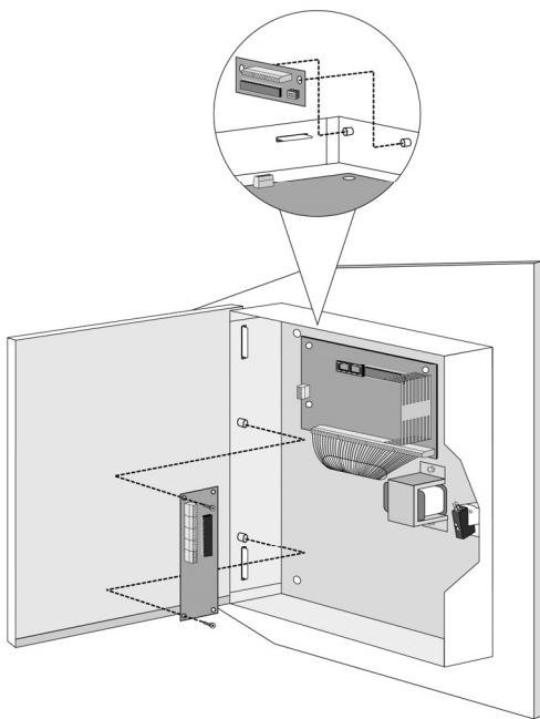
Figura 2-1: Posizionamento della Scheda principale
