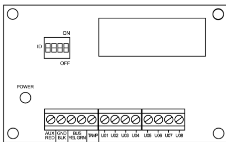
Figura 3-6: Modulo di Esp. Uscite E08
