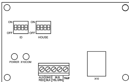
Figura 3-7: Modulo di Esp. Uscite X-10
