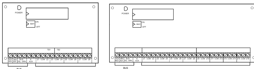
Fig. 3-3: Modulo di Espansione 8 Zone ZE8 Fig. 3-4: Modulo di Espansione 16 zone ZE16
