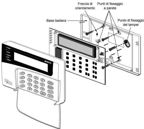
Figura 3-2: Installazione e Vista frontale Tastiera.
